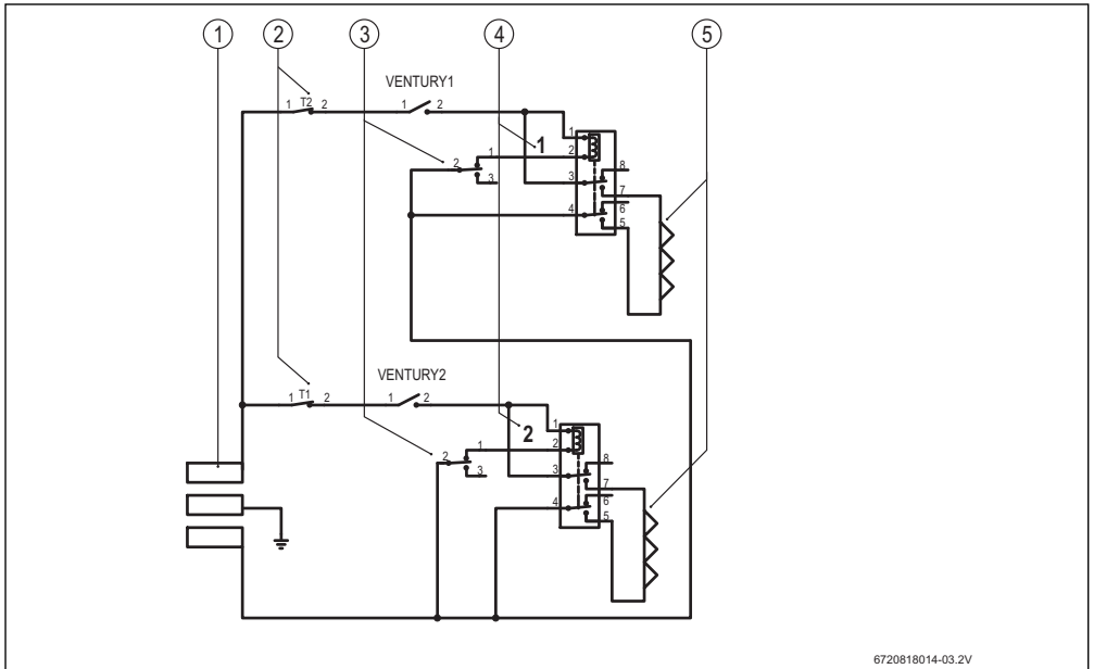
Fig. 4 Esquema interno de conexión 9.5kW
