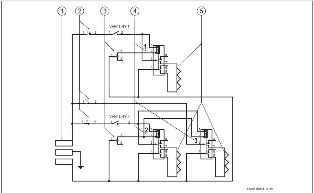
Fig. 5 Esquema interno de conexión 12kW
