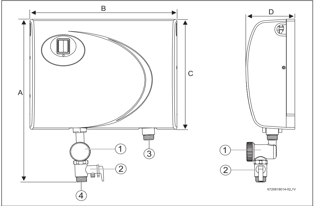
Fig. 3 Dimensiones en mm
