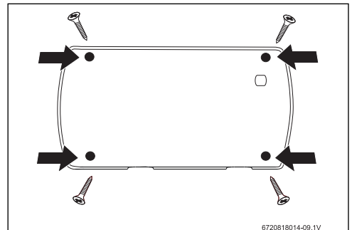
Fig. 20 Orificios de montaje
